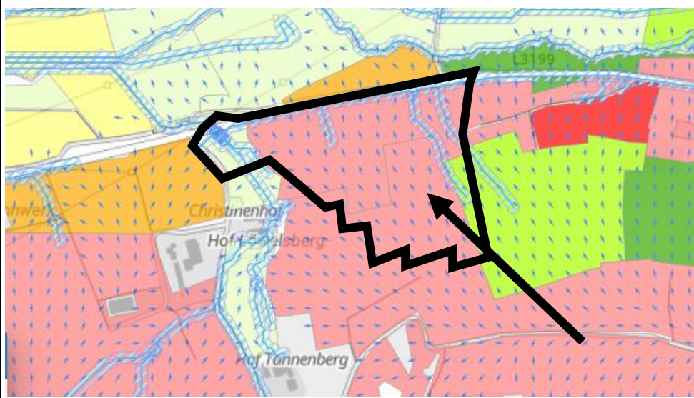
Abb. 15: Fließpfadkarte
