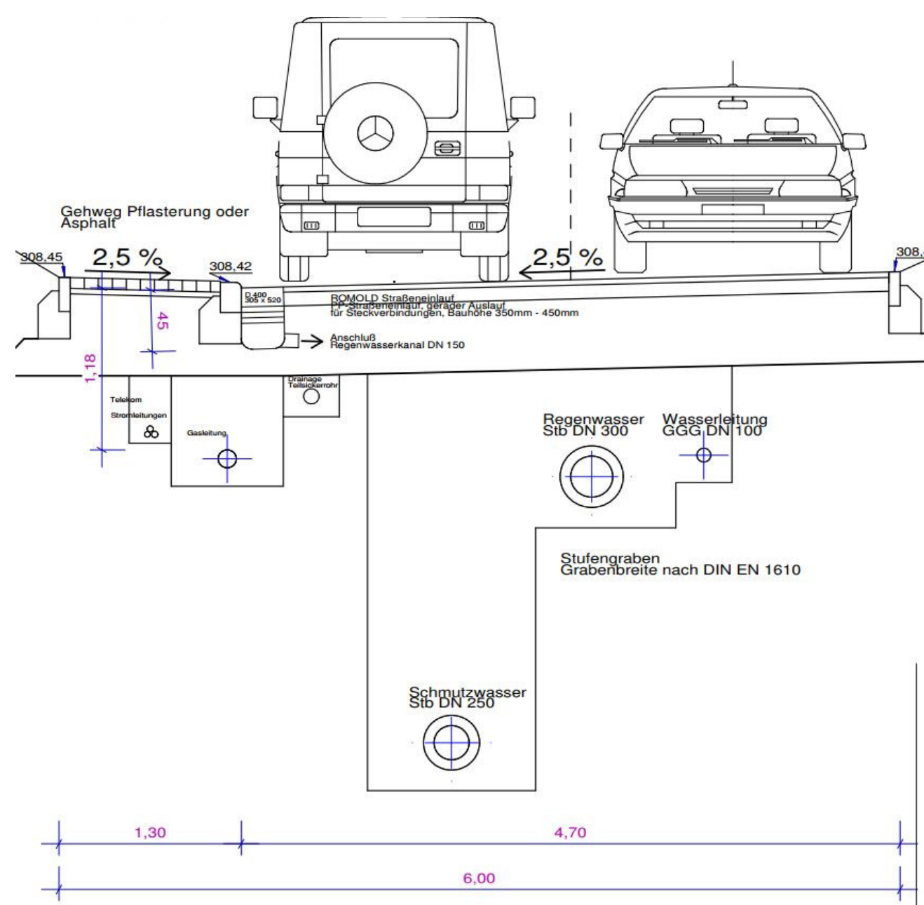
Regelquerschnitt Straße:
