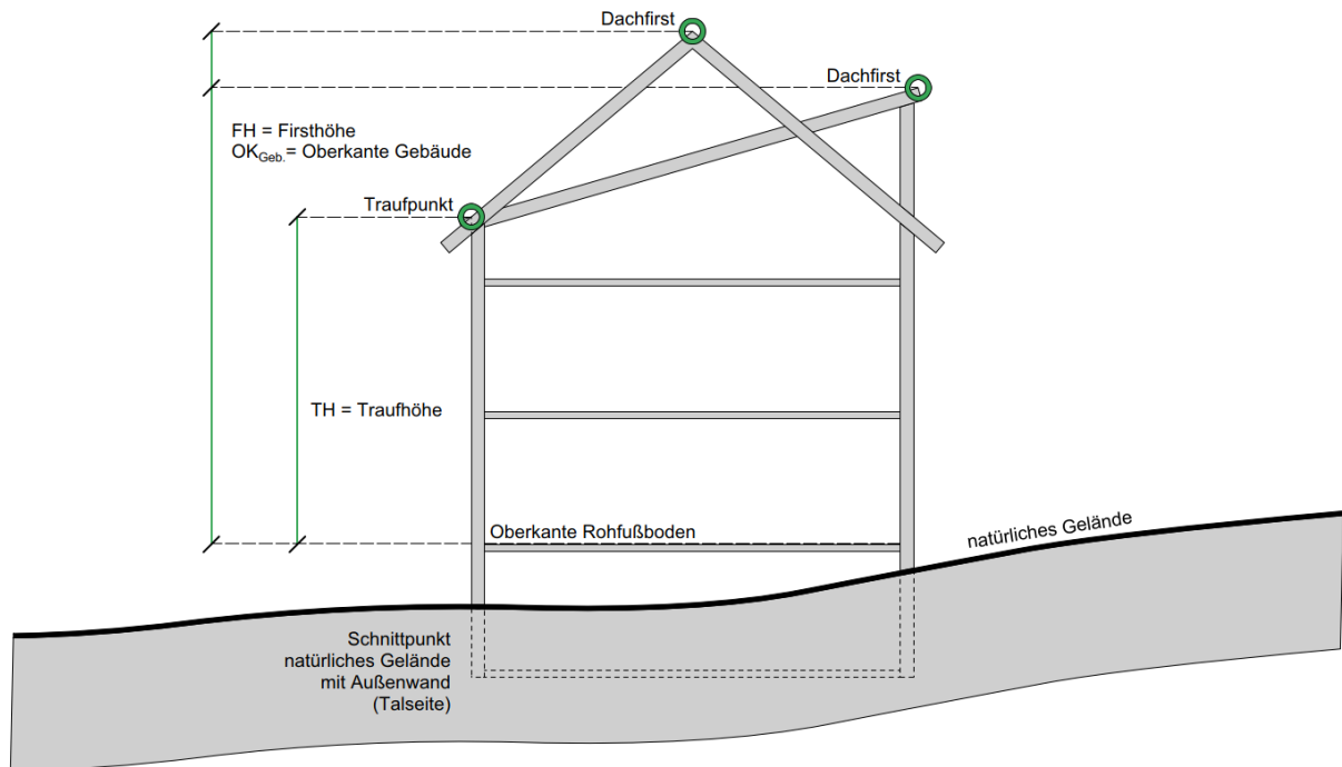
Abb.16: Schematische Darstellung der Höhenentwicklung
