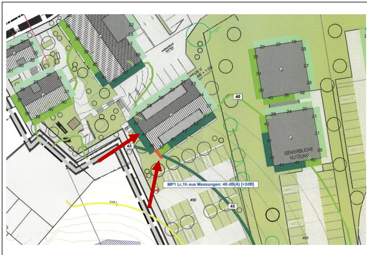
Abb. 20: Geräuschbelastung der geplanten Bebauung, Nachtzeit Isophonendarstellung - 1OG
