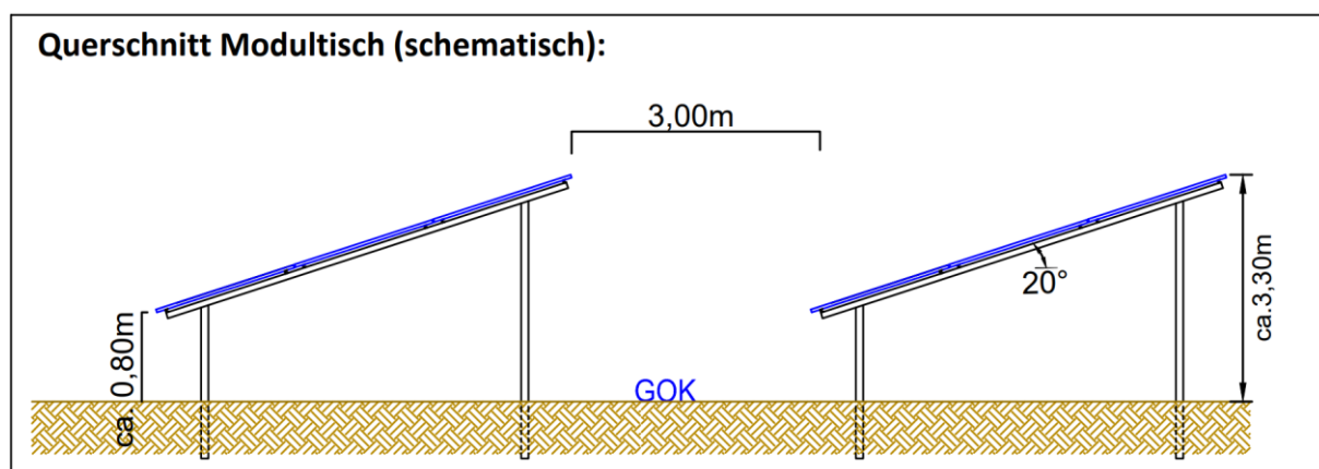
Abbildung 3: Schnittzeichnung - Quelle: Auftraggeber
